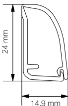
4561 COVER(IT) Wandleiste, selbstklebend für Wand.
