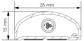
4545 COVER(IT) Wandleiste, selbstklebend für Wand.
