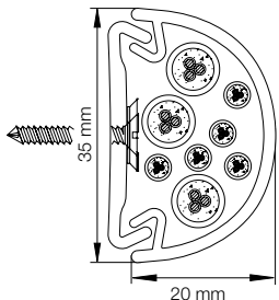
4170 COVER(IT) Wandleiste zur Abdeckung von vom Boden nach oben führenden Leitungen, z. B. zu wandmontiertem TV.
