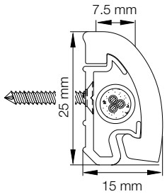
4170 COVER(IT) Wandleiste zur Abdeckung von vom Boden nach oben führenden Leitungen, z. B. zu wandmontiertem TV.
